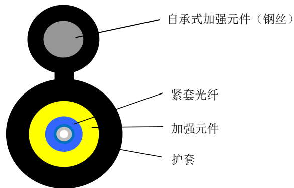
自承式圆形引入光缆
